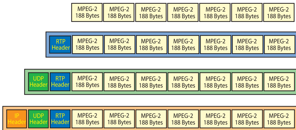
Abbildung 3.5: Verarbeitung der MPEG-2 TS-Pakete
